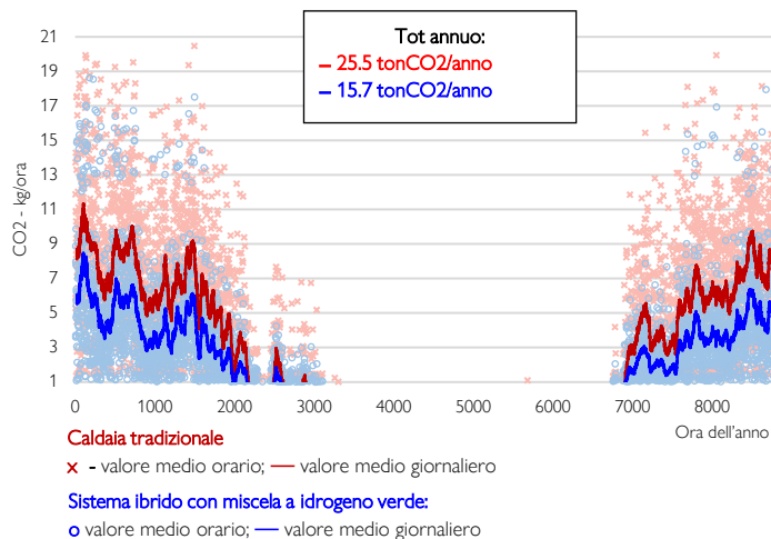
Figura 5-17. Profili di emissione medi orari e medi giornalieri di un sistema ibrido alimentato a idrogeno “verde” rispetto ad una caldaia tradizionale nel caso di un condominio in zona E
