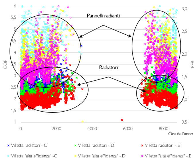
Figura 5-16. Esempi di risultati di simulazioni dinamiche, in termini di prestazioni orarie di una pompa di calore elettrica aria-acqua (coefficiente di prestazione COP e Primary Energy Ratio PER) a seconda della zona climatica, del tipo di edificio e dei terminali di impianto
