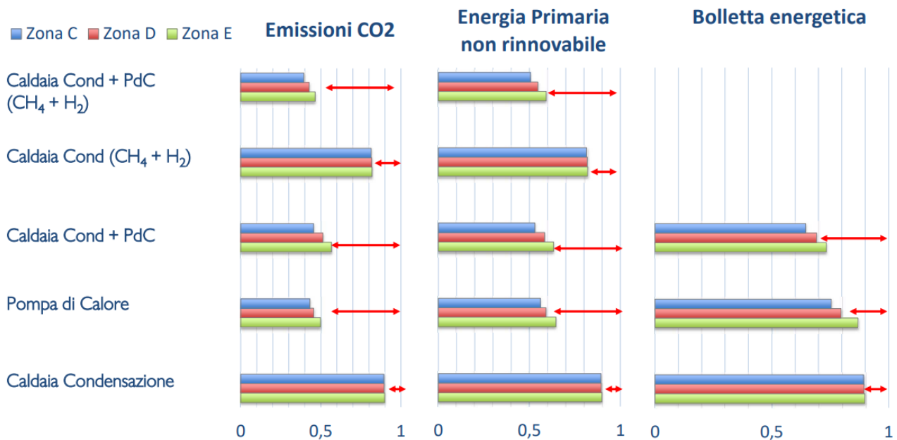
Figura 5-18. Prestazioni ottenibili attraverso l'utilizzo delle diverse tecnologie di riscaldamento
